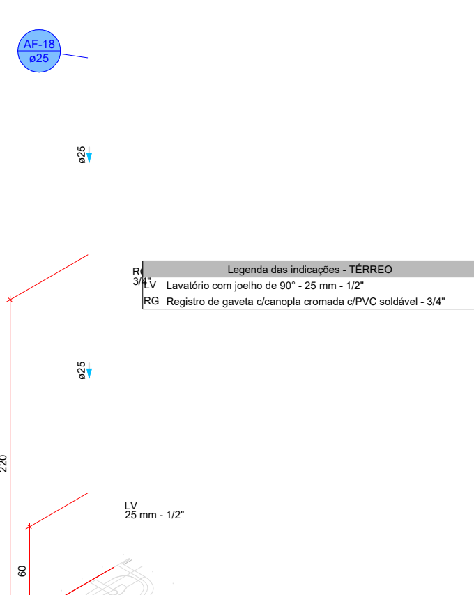
DETALHE HID-18 1:25
