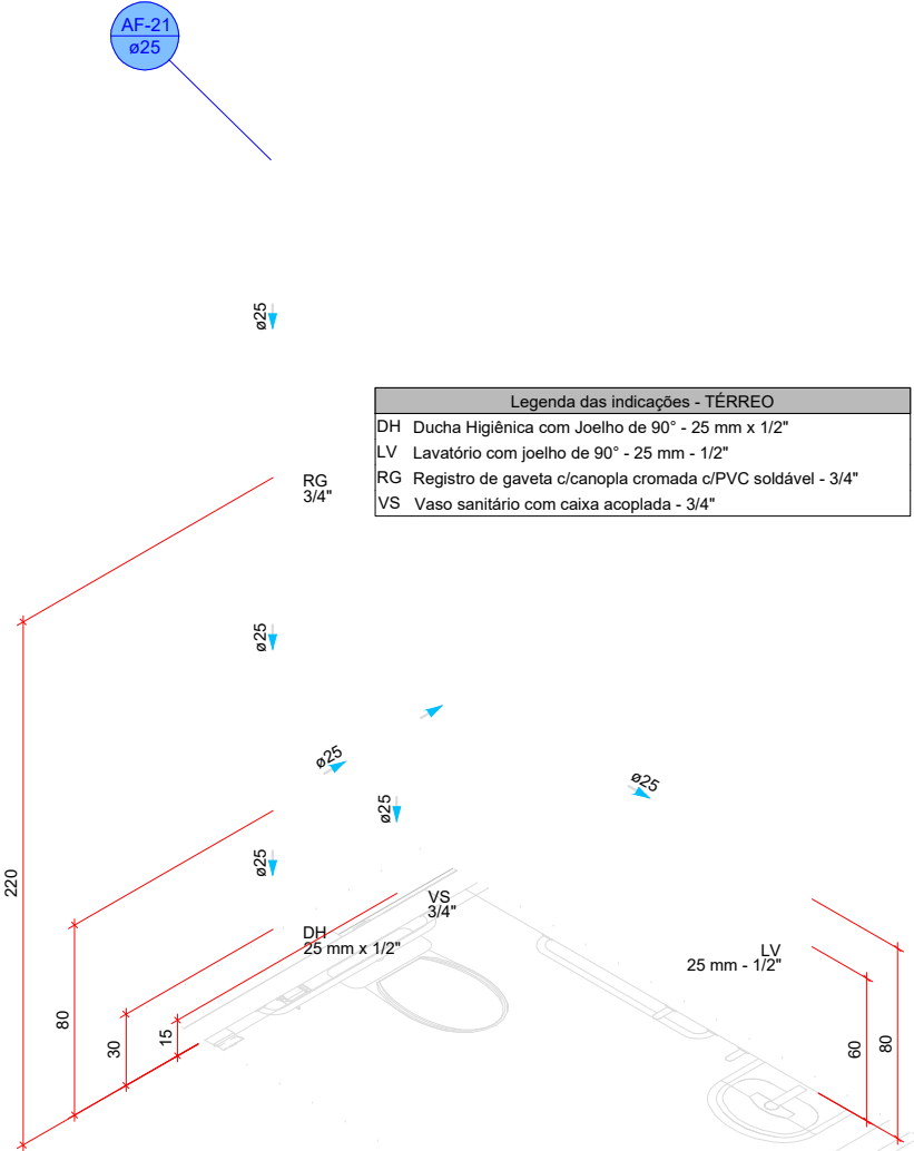
DETALHE HID-21 1:25
