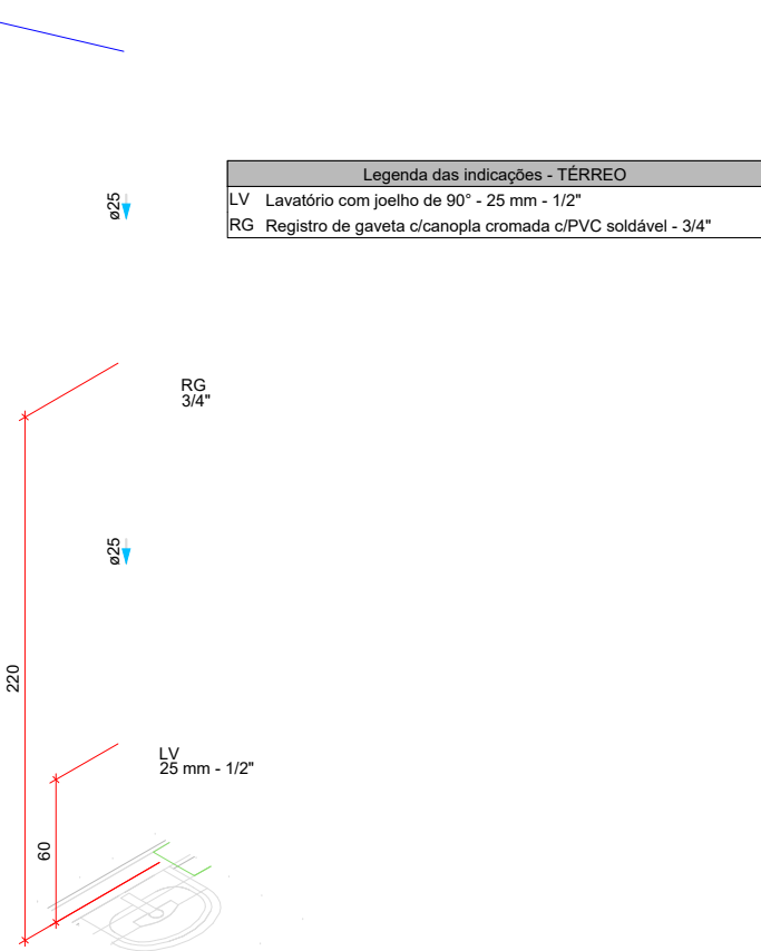
DETALHE HID-15 1:25
