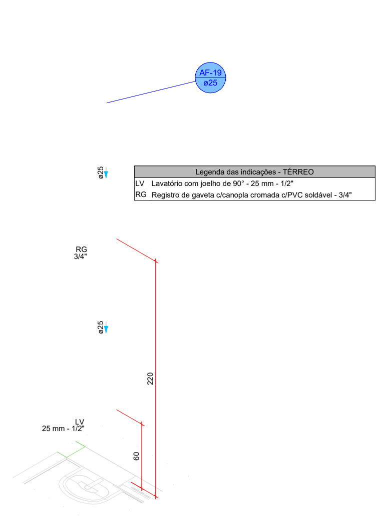
DETALHE HID-20 1:25
