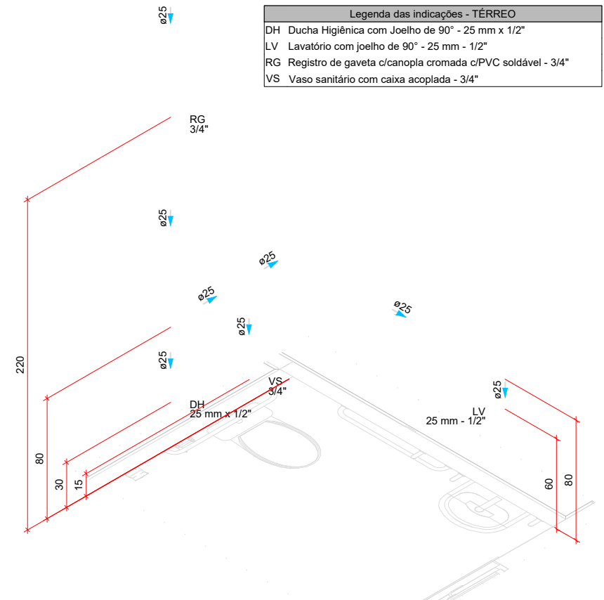
DETALHE HID-17 1:25
