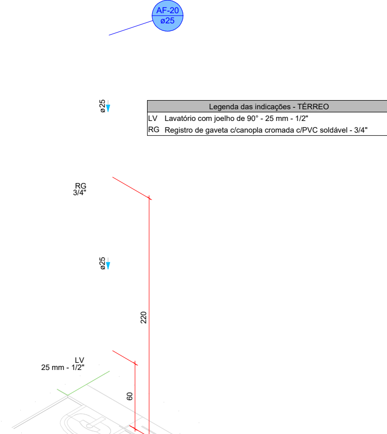
DETALHE HID-19 1:25
