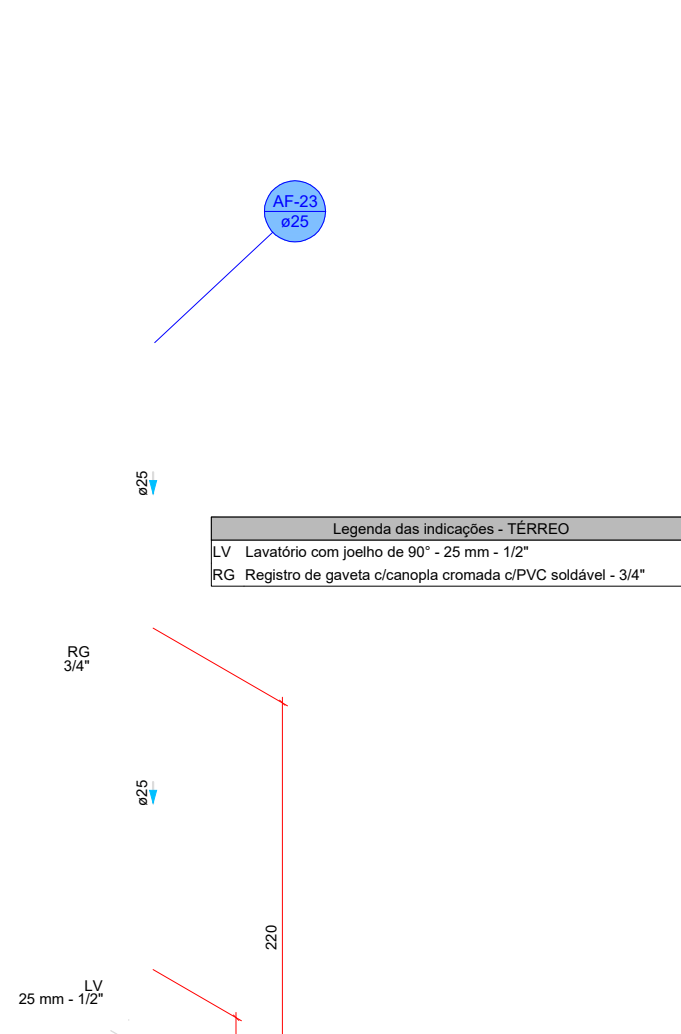
DETALHE HID-23 1:25
