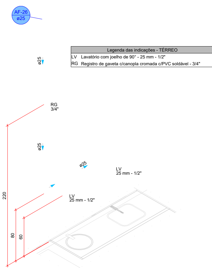
DETALHE HID-25 1:25
