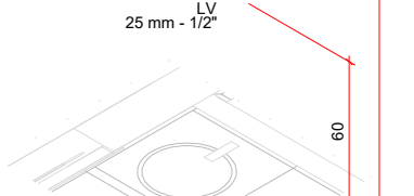
DETALHE HID-9 1:25
