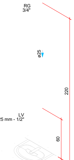
DETALHE HID-7 1:25
