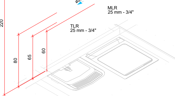
DETALHE HID-6 1:25
