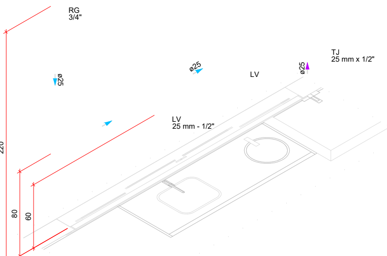
DETALHE HID-11 1:25
