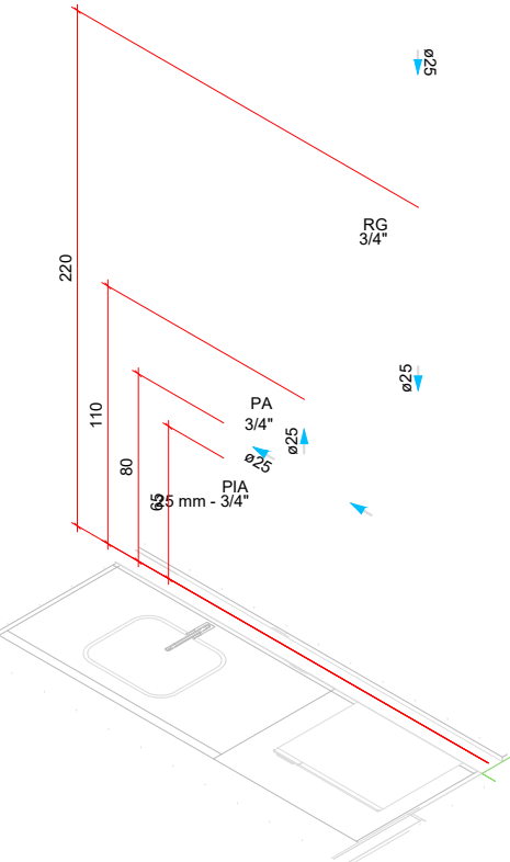
DETALHE HID-3 1:25
