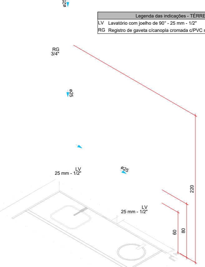
DETALHE HID-10 1:25
