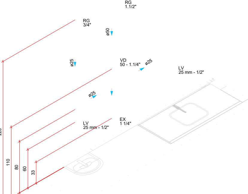
DETALHE HID-8 1:25
