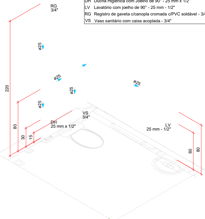
DETALHE HID-12 1:25
