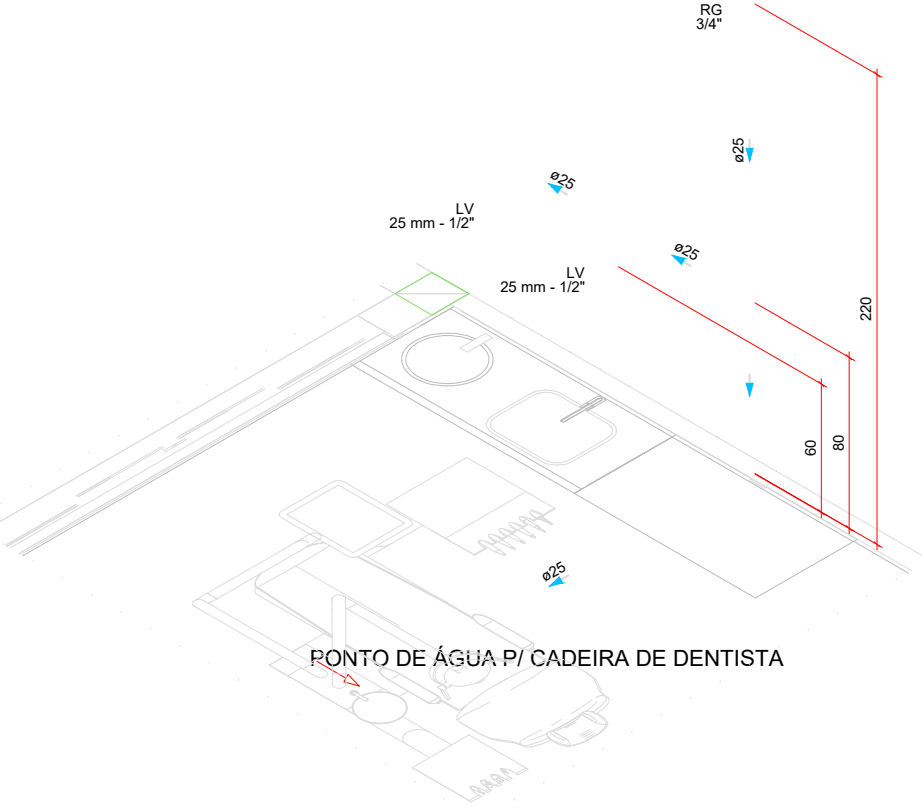
DETALHE HID-13 1:25
