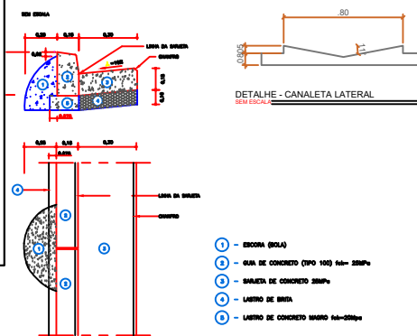
DETALHE DE GUIA E SARJETA
